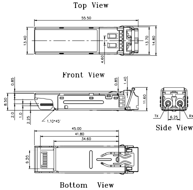
OPN-SG161-D39LC2
