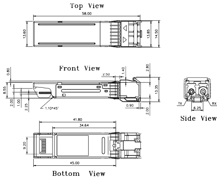
OPN-SG161-D39LC2I
