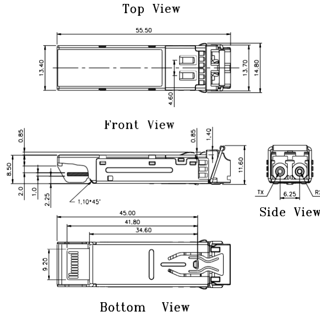
OPN-SG153-D19LC2
